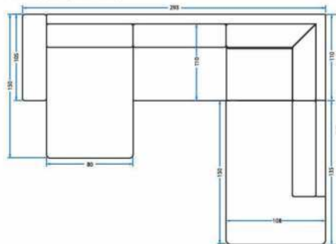
Visão Superior (Retrátil Aberto)
