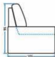
Visão Lateral (Módulo)
